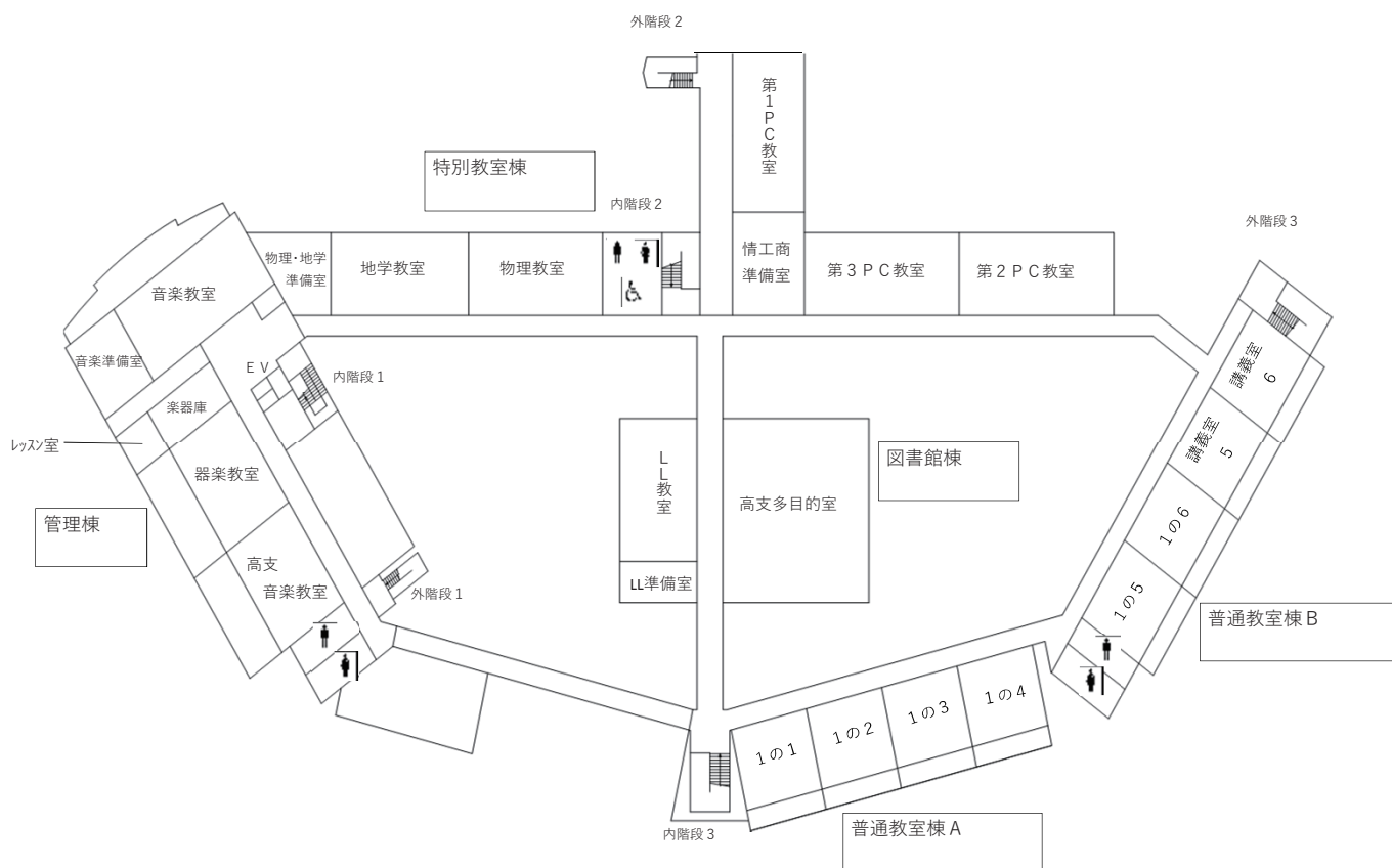
4 階平面図
